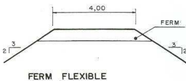
SECCIÓ B-B
